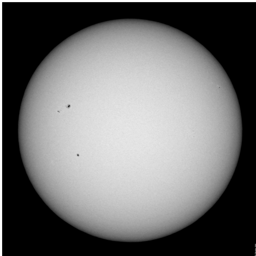
Figura 6- Sol (20051213) num período de menor actividade. Takahashi FS128 F/8.1 + Canon 300D. Prisma Herschel Baader. Pedro Ré (2005).
