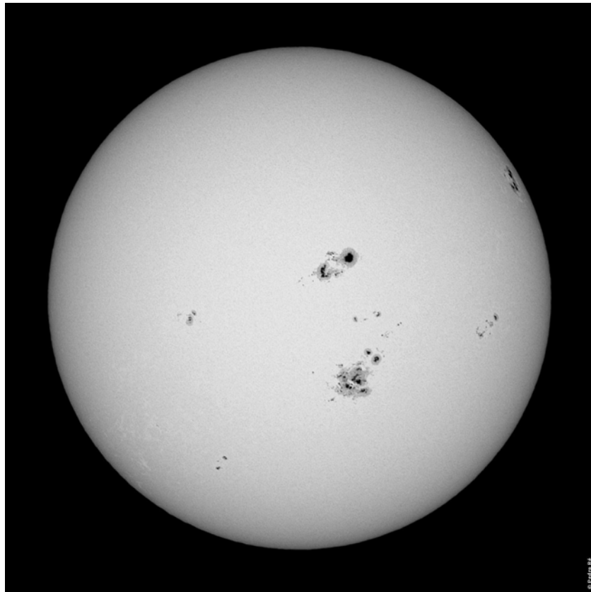
Figura 5- Sol (20031029) num período de grande actividade. Takahashi FS128 F/8.1 (VR-1) + Fuji FinePix S1 Pro. Filtro Frontal Baader. Pedro Ré (2003).
