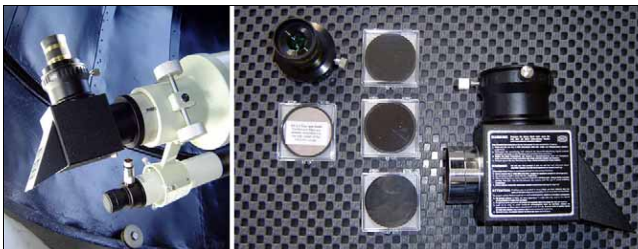
Figura 1- Prisma Herschel Baader. Pedro Ré (2005).
