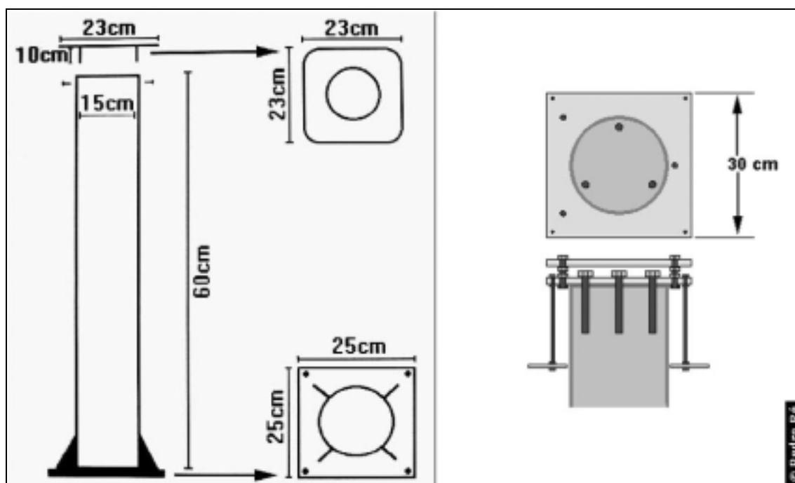
Figura 4- Dois projectos de pilares.
